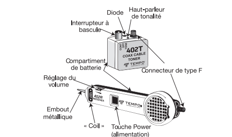
Fig. 1 - Commandes
