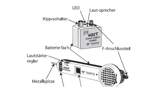
Abb. 1 - Regler
